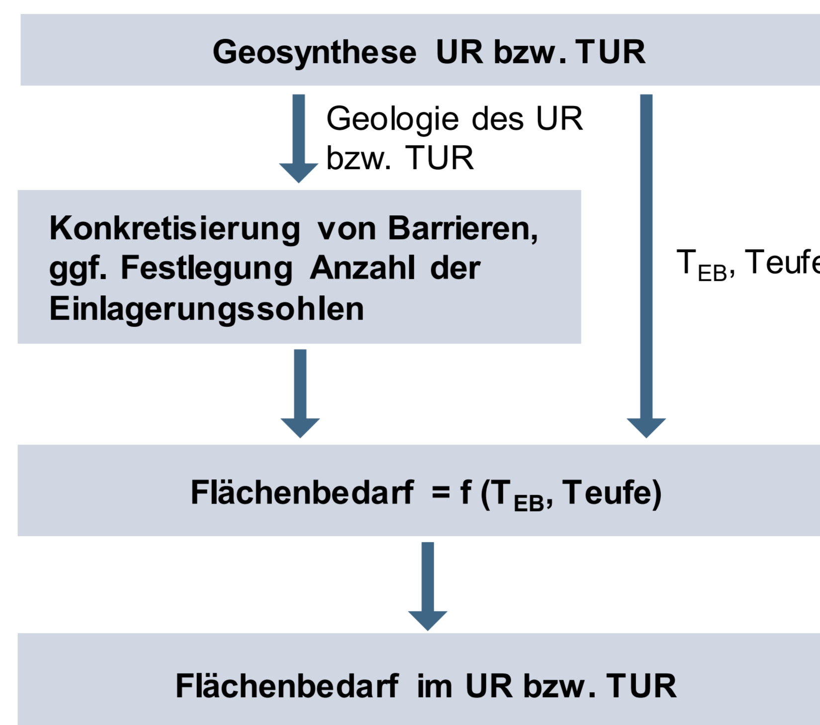
Abb. 2: Schematische Darstellung der Methodik zur (teil-)untersuchungsraumspezifischen vorläufigen Endlagerauslegung im Rahmen der rvSU (Teil 2 der Methodik), (Quelle: BGE)
